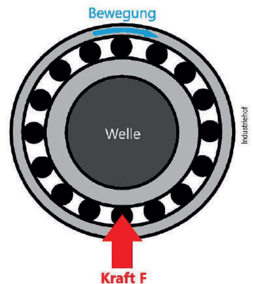
Seitenansicht eines Kugellagers. Der Innenring hat die Punktlast und der Außenring die Umfangslast.
